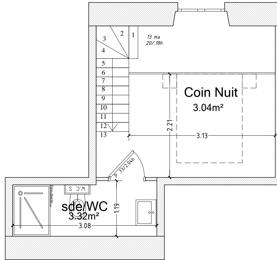
Niveau 2 mezzanine
